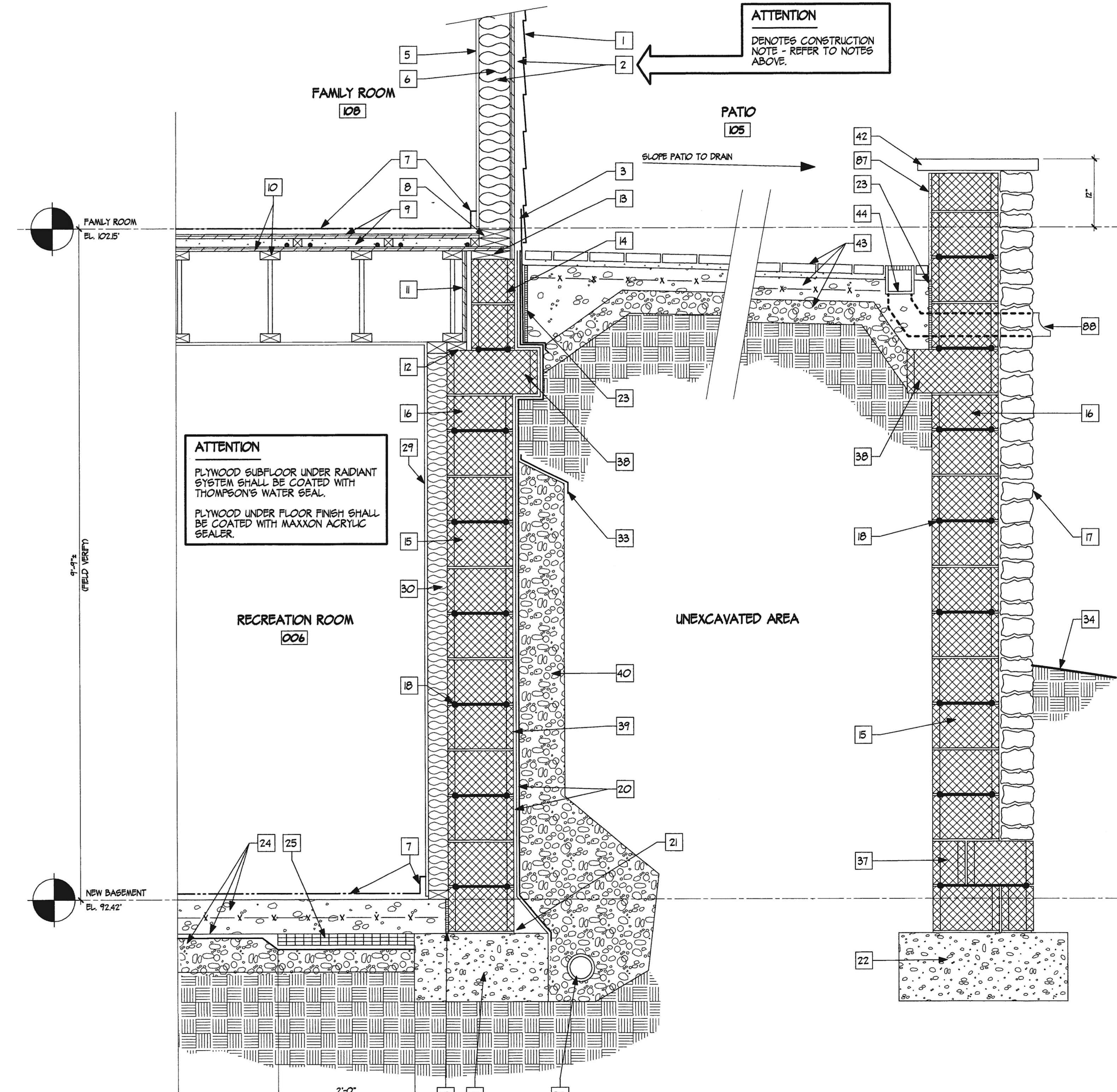
DETAIL O SCALE: 1/4"=1'-0"
