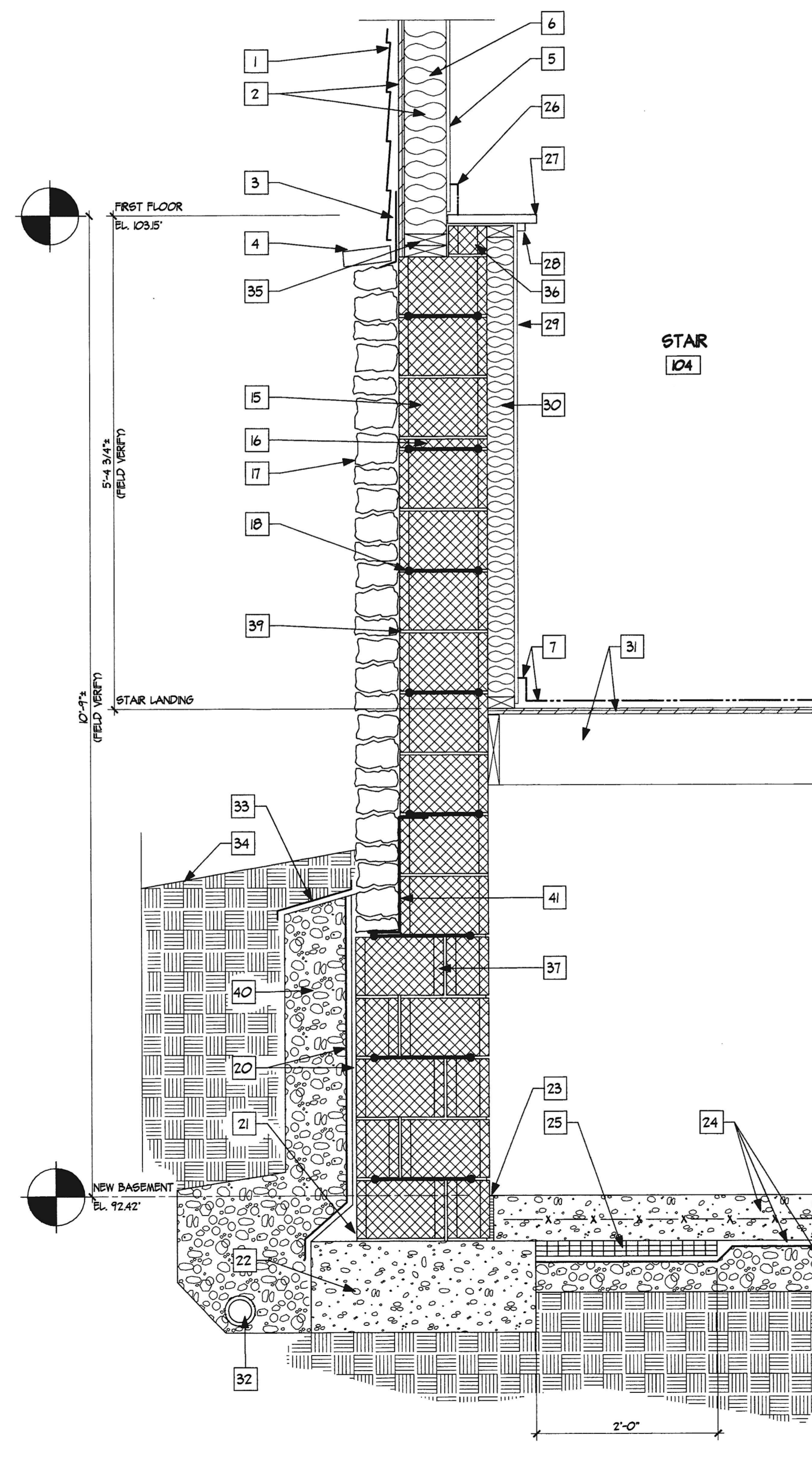
DETAIL N SCALE: 1/4"=1'-0"
