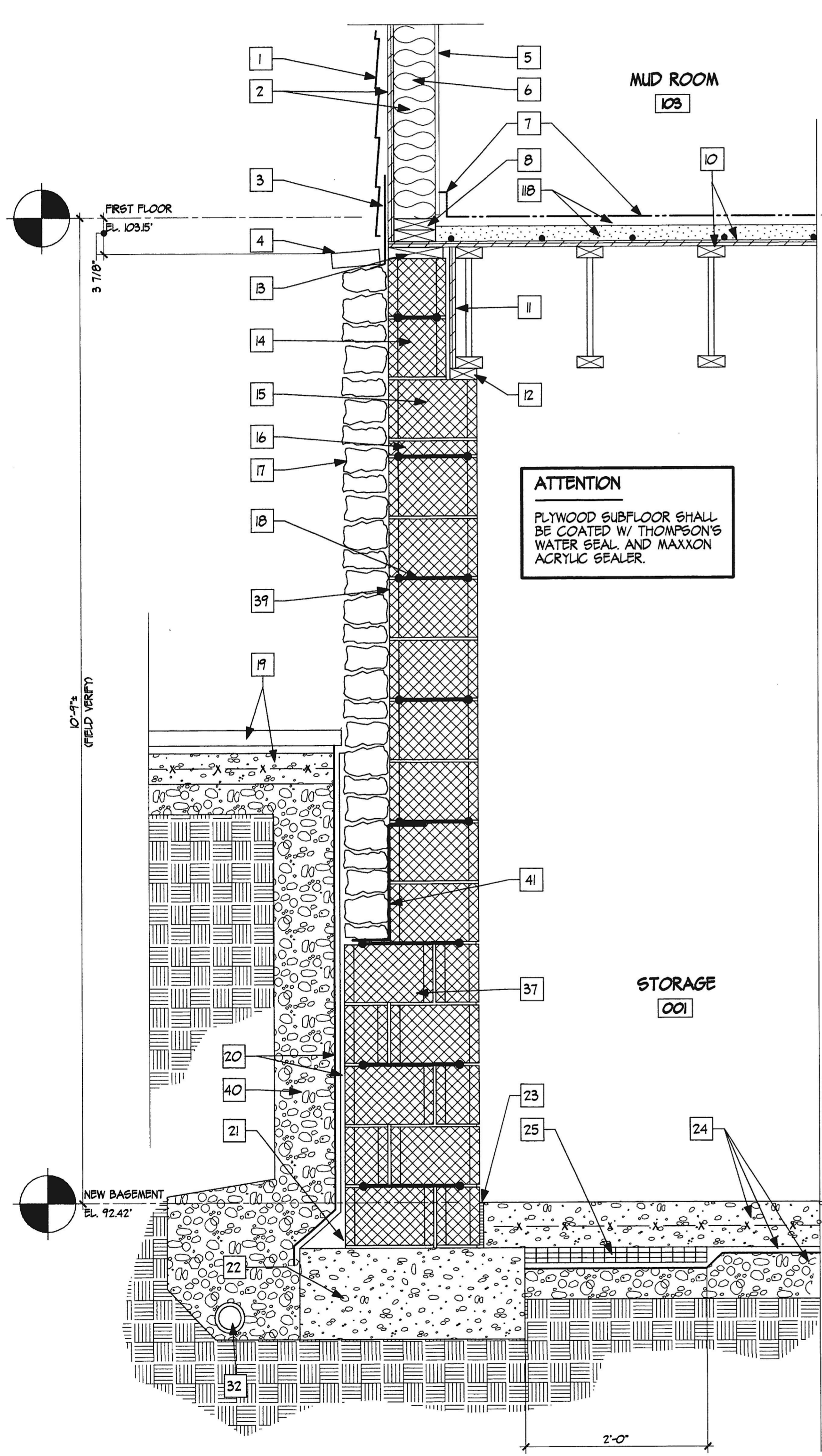
DETAIL M SCALE: 1/4"=1'-0"
