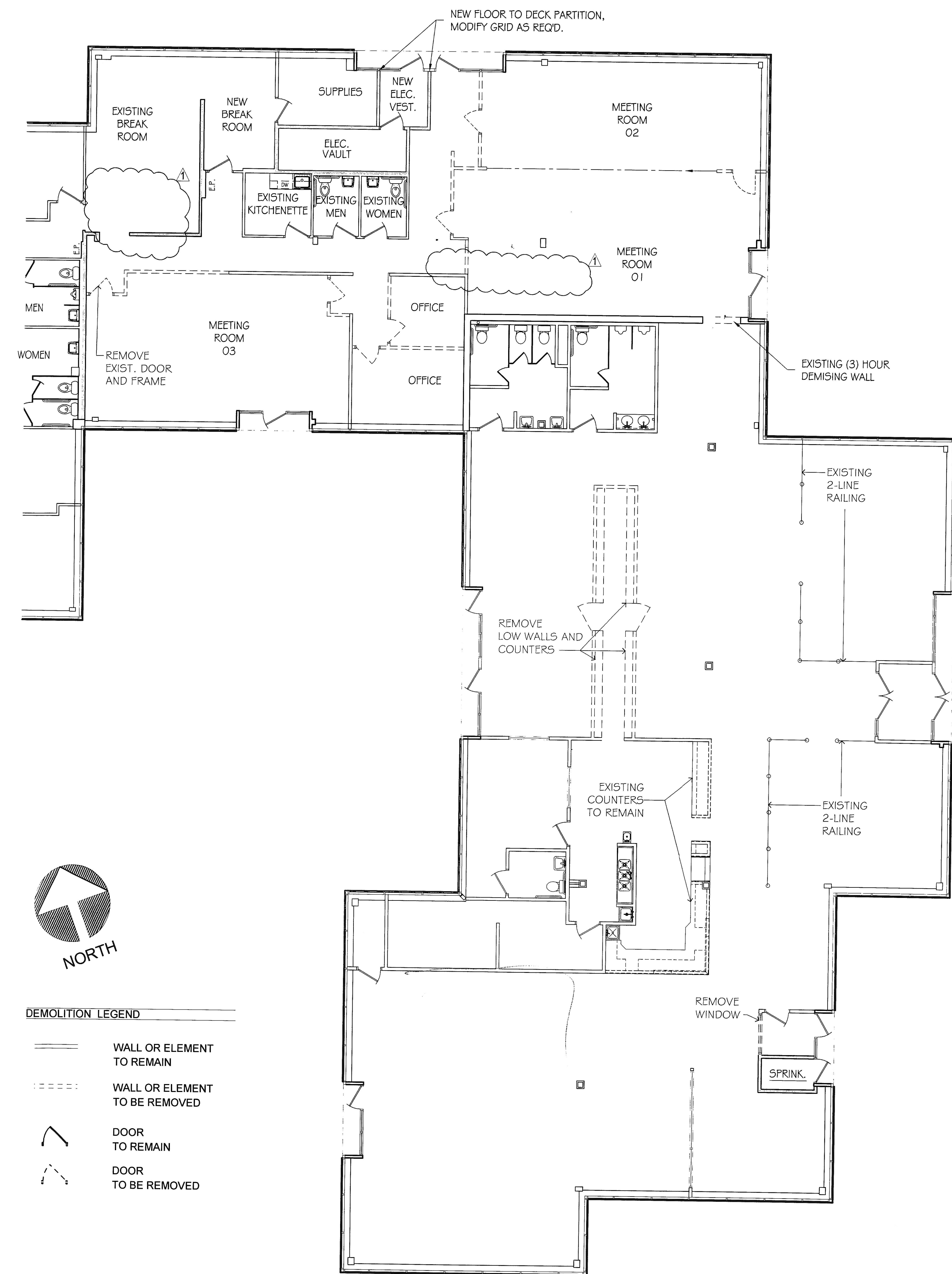
2 DEMOLITION PLAN Scale: 1/8" = 1'-0"
