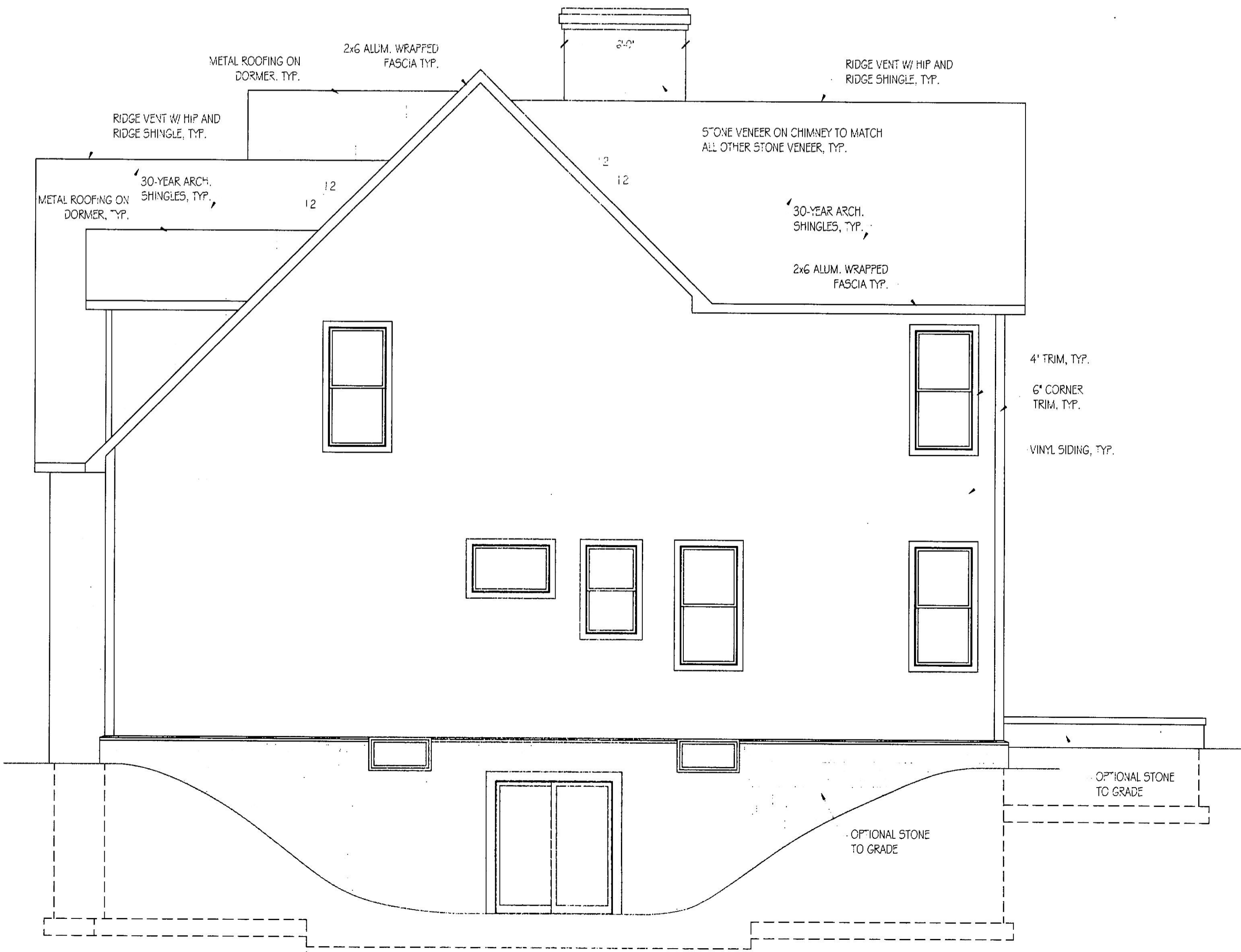
RIGHT ELEVATION SCALE: 1/4" = 1'-0"
