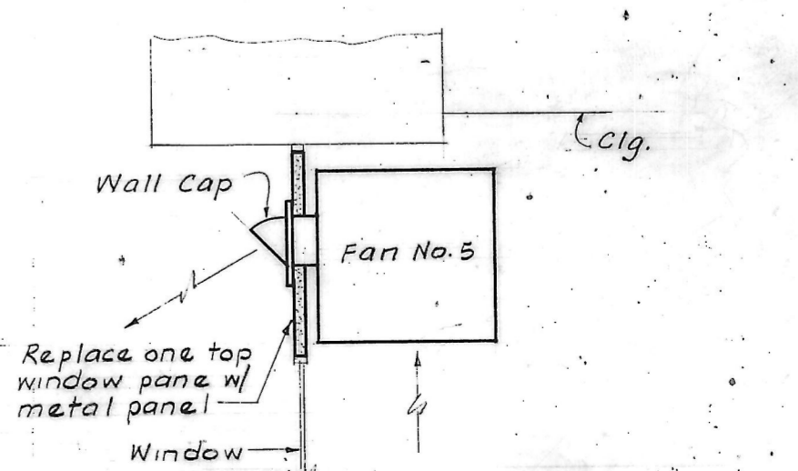
SECTION MIP9 Scale: 1" = 1'-0"
