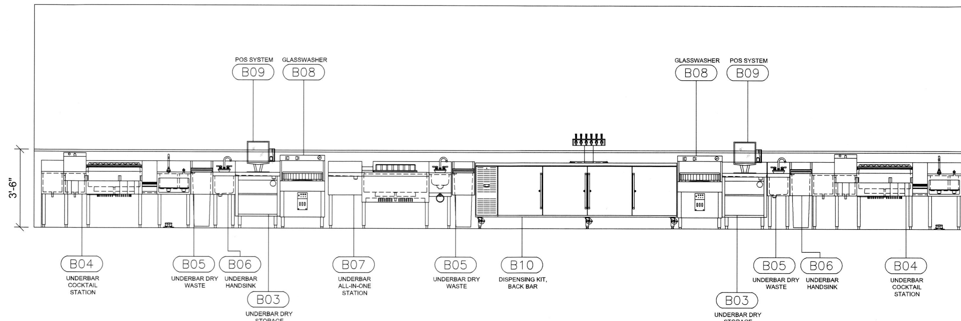
1 BAR SCALE: 3/8" = 1'-0"
